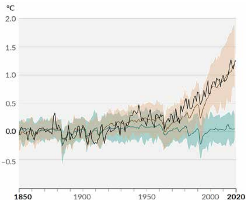
Figura 1: Temperaturas medias de la superficie de 1850 a 2020. La curva en negro representa las temperaturas observadas. Las curvas en color representan las simulaciones numéricas de la temperatura: en azul sin actividades humanas y en marrón con.
